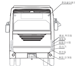
<후면도>
