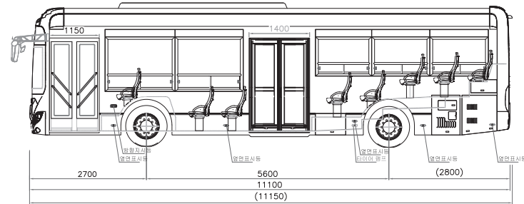
<우측면도>
