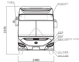
<정면도>
